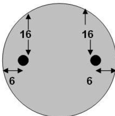
Εικόνα A-4. Αποστάσεις Ακίδων στο Οπίσθιο Μέρος του Μεταλλικού Διακριτικού
