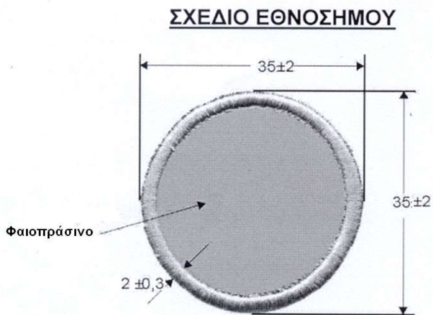
Διαστάσεις βάσης κέντησης εθνοσήμου και ενισχυτικού κεντήματος
